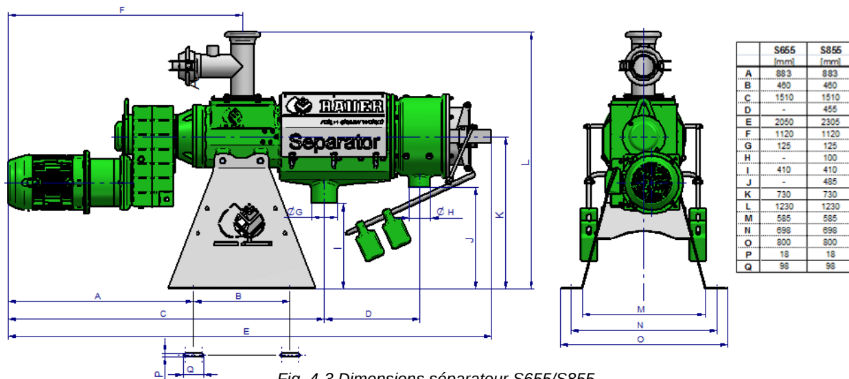
Fig. 4-3 Dimensions séparateur S655/S855
