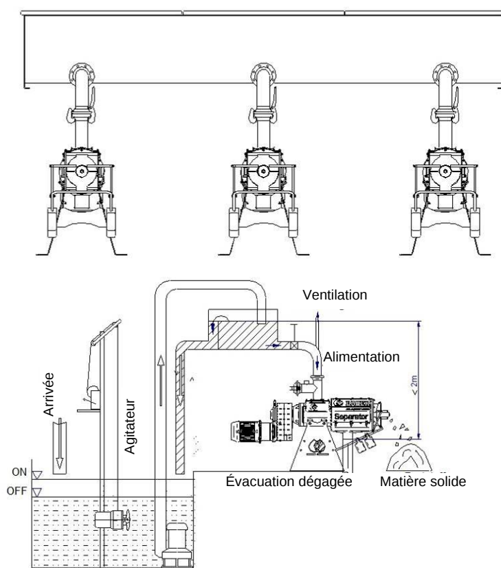
Fig. 9-1. Disposition typique de 3 séparateurs utilisés en parallèle
