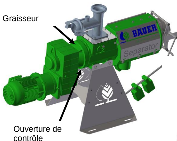
Fig. 13-1 Traitement avec liquide de blocage
