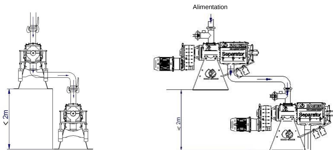
Fig. 10-1 Disposition typique de 2 séparateurs en série
