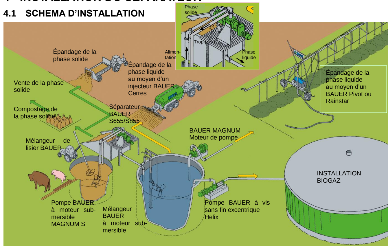
Fig. 4-1 Schéma d'installation
