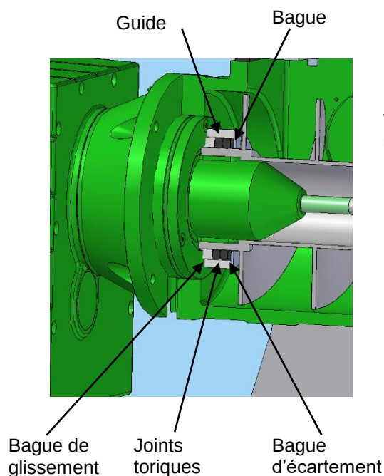
Fig.13-4 Joint supplémentaire
