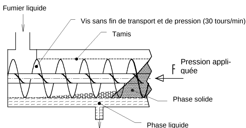
Fig. 3-1 Description des fonctions
