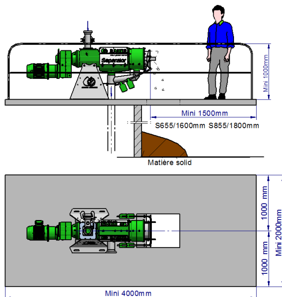
Fig. 4-4 Dimensionnement du lieu d'installation
