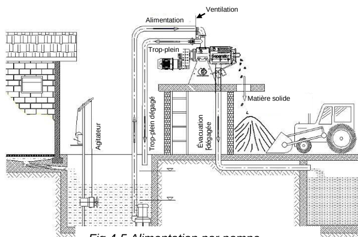
Fig.4-5 Alimentation par pompe
