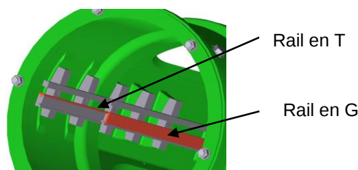
Fig. 13-7 Carter du séparateur S855 avec les rails de guidage du tamis et les profils en G pour tamis standard dans la partie drainage et profil en T pour tamis HD dans la partie compactage
