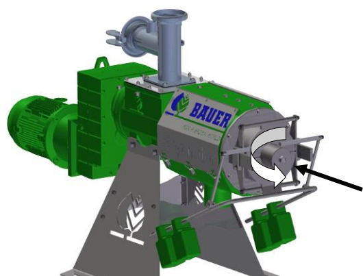
Fig. 5-1 Sens de rotation de la vis sans fin
