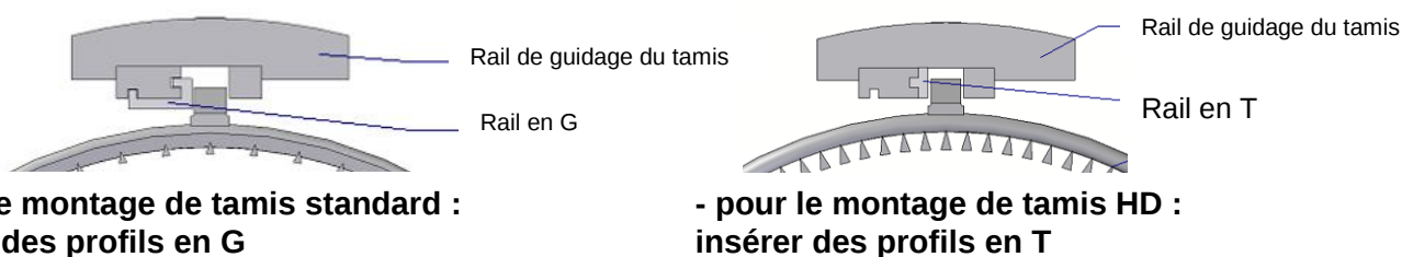
Fig. 13-6 Rail en G -- Rail en T
