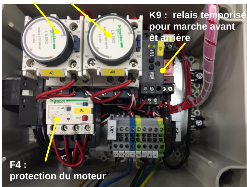
Fig. 15-2 Commande
