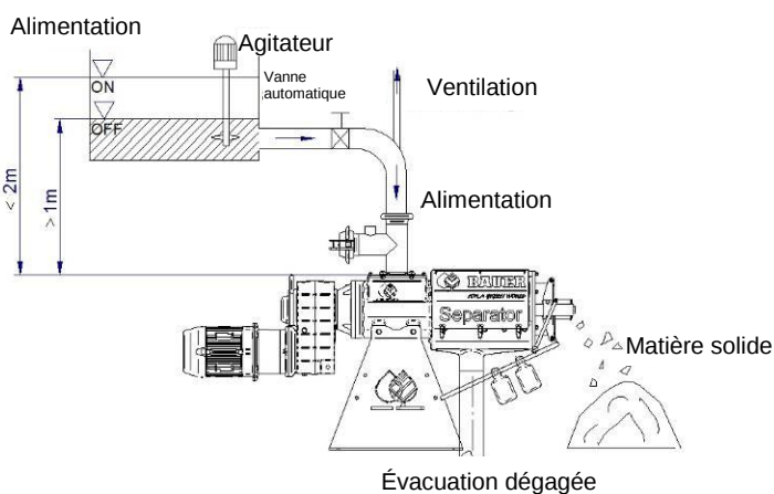
Fig.4-6 Alimentation par la gravité depuis un réservoir surélevé
