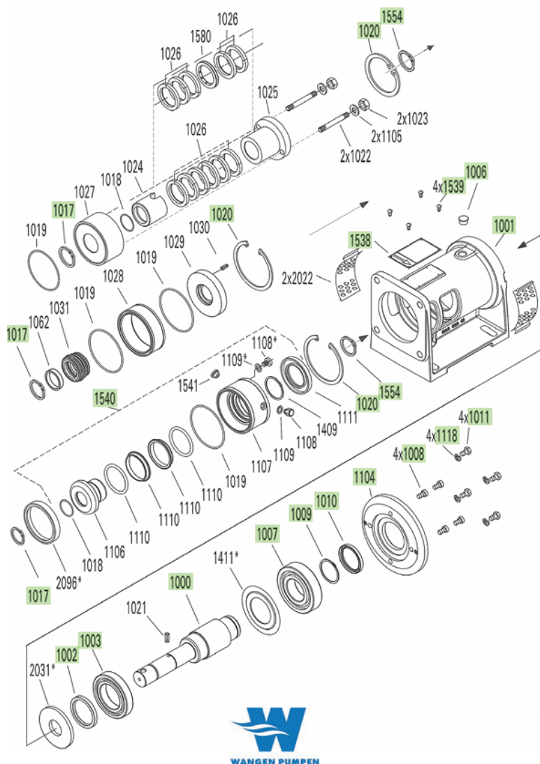
Éclaté support de palier KL 50
